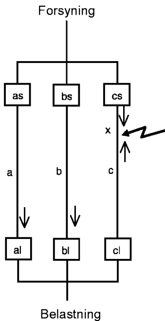
Fig. A.3 Strømførløb ved fejls opståen.
