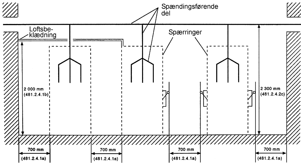
Fig. 48A - Betjenings- og vedligeholdsgange i installationer med beskyttelse ved spæringer
