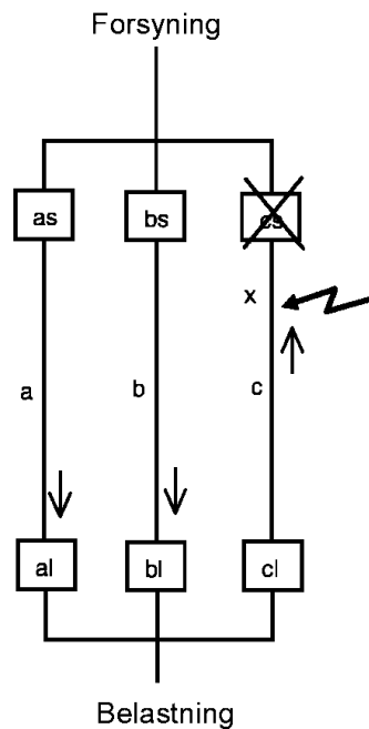
Fig. A.4 Strømførløb efter udløsning af beskyttelsesudstyret cs.
