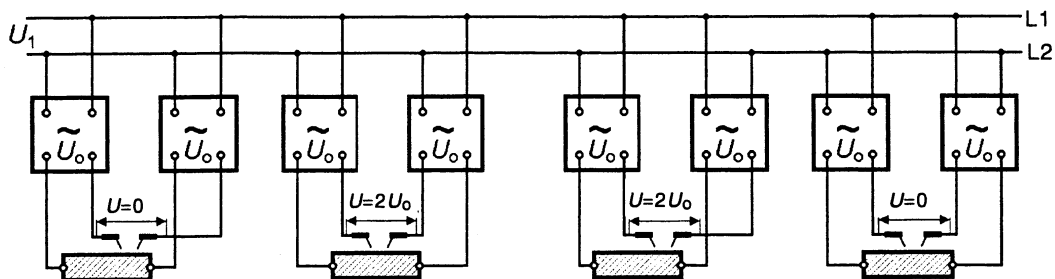
Fig. 812B – Eksempel på vekselspænding mellem elektrodeholdere eller brændere- Enfaset forsyning fra de samme to faser i en trefaset forsyning
